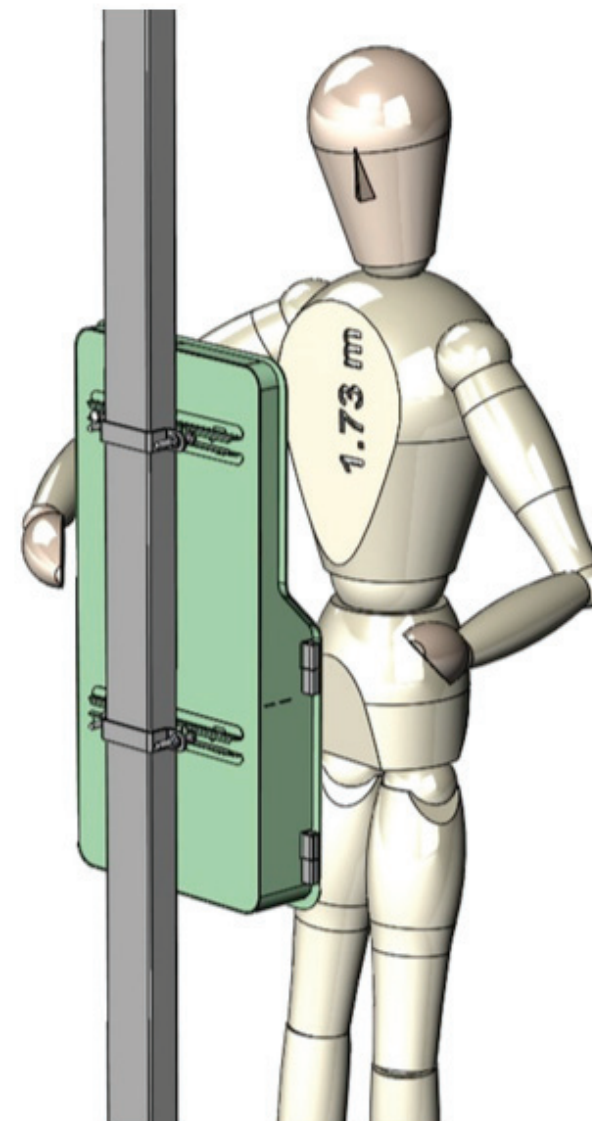
Exemple de fixation poteaux (non fournis)
